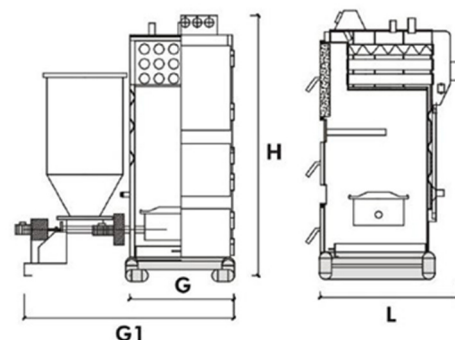
Atmosfere çıkan baca gazı sıcaklığından maksimum faydayı sağlayan 4 geçişli ve sulubazlı sistem
